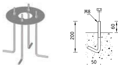
Комплект анкерных болтов АВ 217. Код заказа — 40217.
