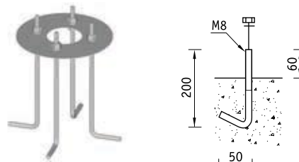
Комплект анкерных болтов АВ 217. Код заказа — 40217.
