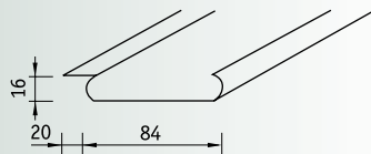
Схема рейки.
